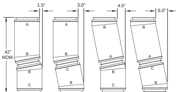
FIG. 28 - VOK CONFIGURATIONS
